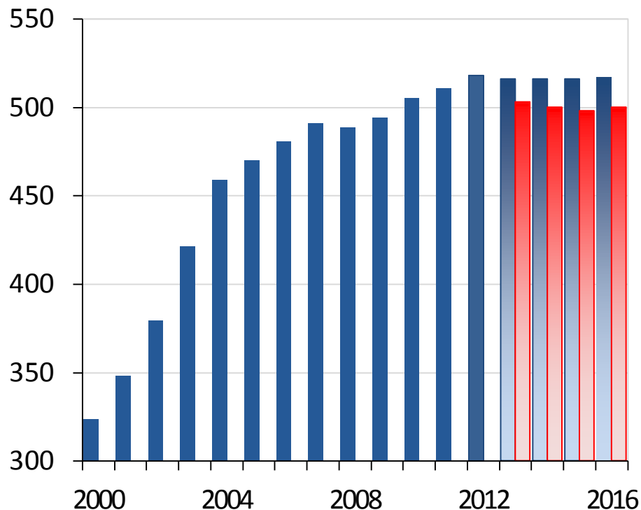
Динамика добычи нефти в 2000-2012 и прогноз до 2016, млн. тонн
