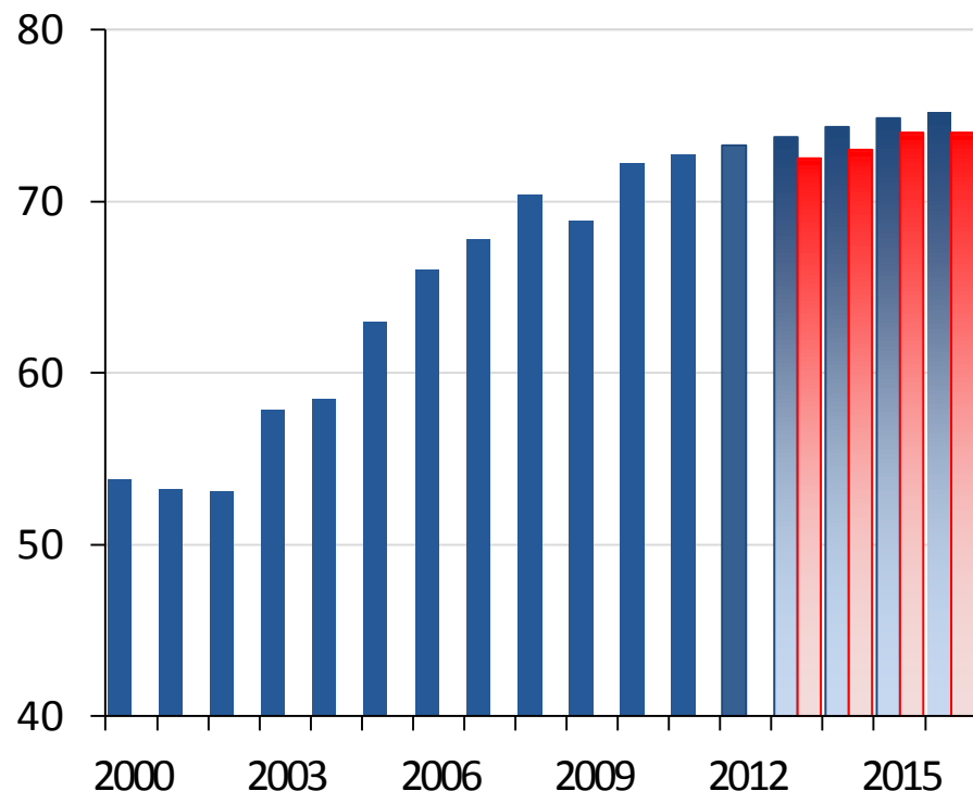
Динамика переработки газа в 2000-2012 и прогноз до 2016, млрд. куб. м
