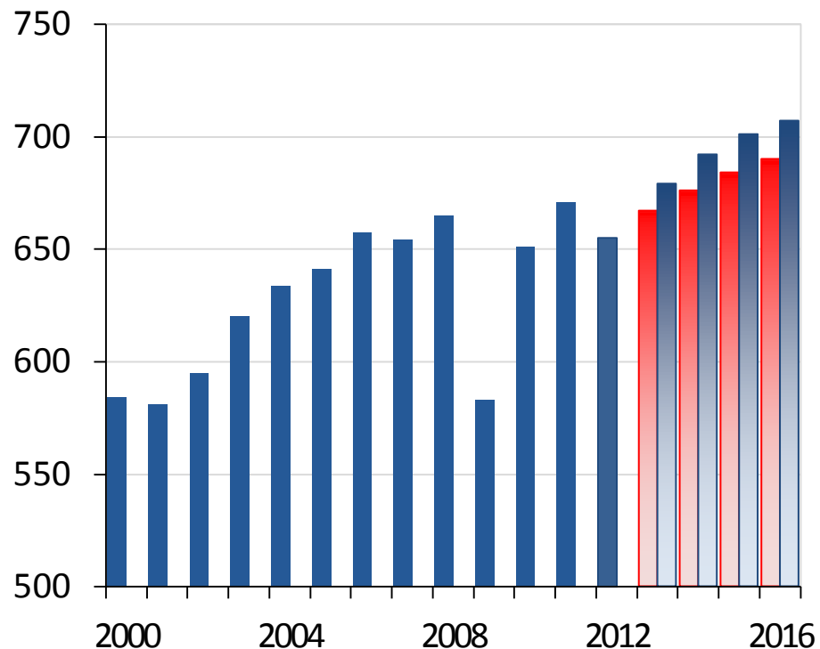
Динамика добычи газа в 2000-2012 и прогноз до 2016, млрд. куб. м
