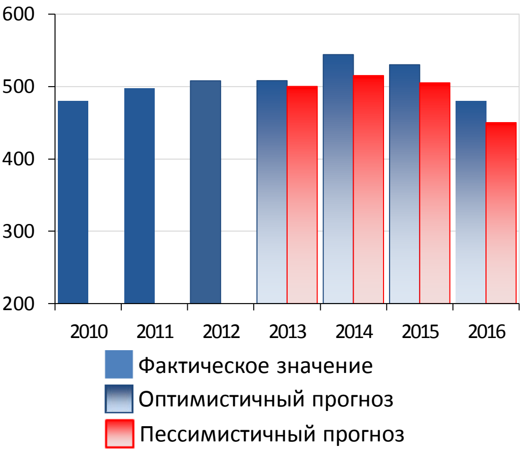
Динамика инвестиций в транспортировку углеводородов и прогноз до 2016, млрд. руб.
