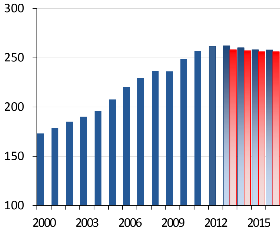
Динамика переработки нефти в 2000-2012 и прогноз до 2016, млн. тонн
